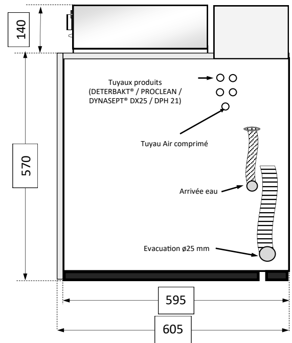
Vue de Côté : Tiroir fermé
